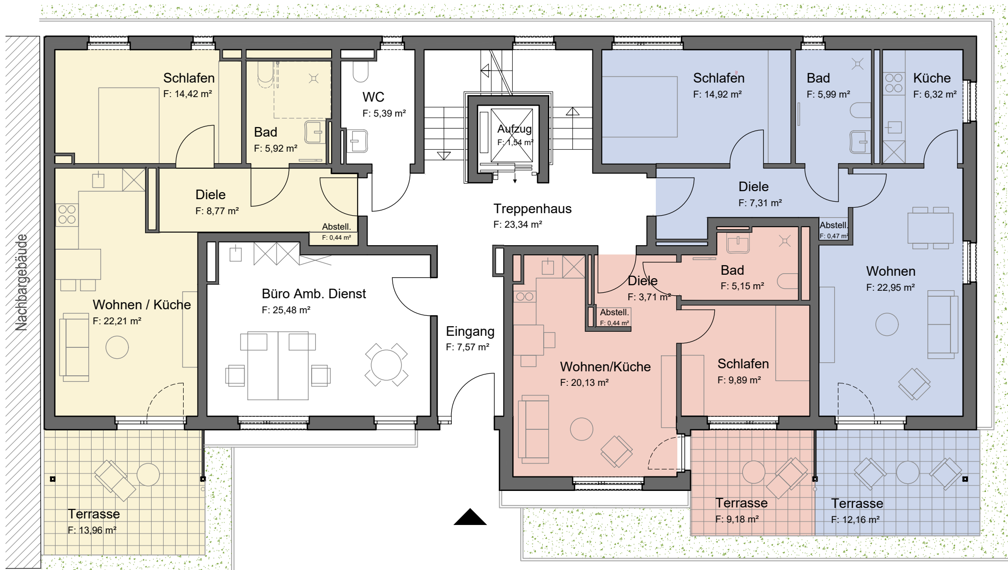
Grundriss Erdgeschoss
